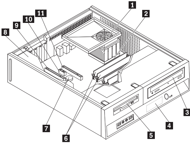
圖 3. 元件位置
