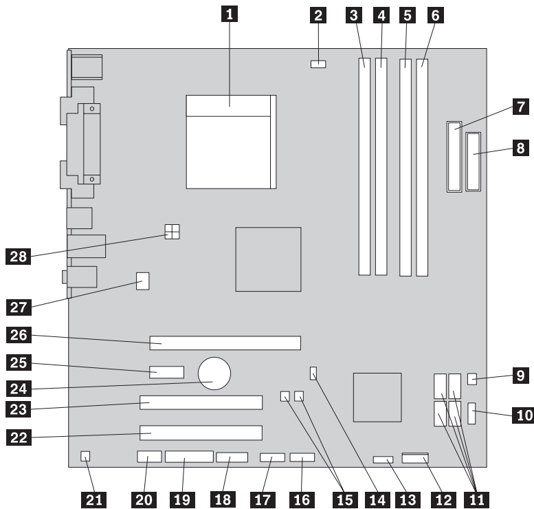
圖 4. 系統主機板零件位置
