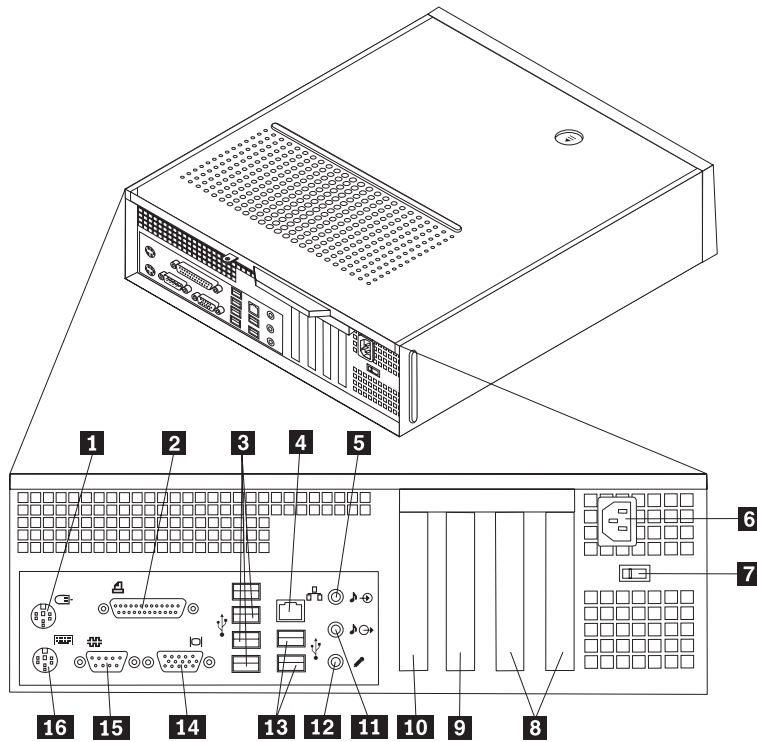
圖 2. 接頭位置
