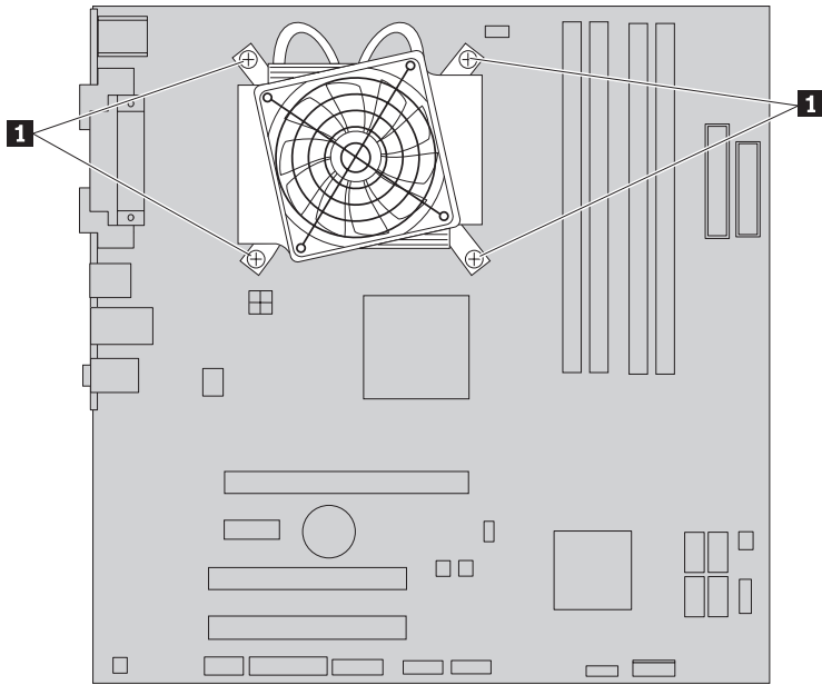
圖 31. 更換散熱器及風扇組件的螺絲
