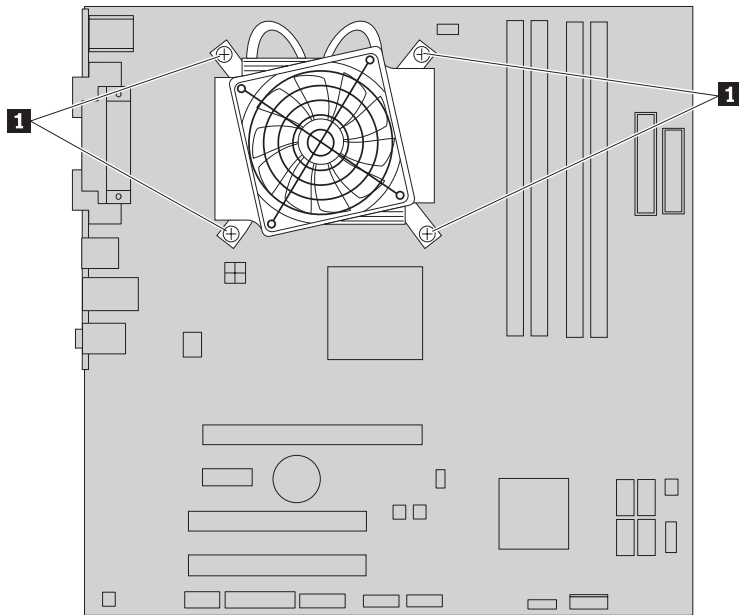
圖 30. 卸下列用螺絲固定的散熱器
