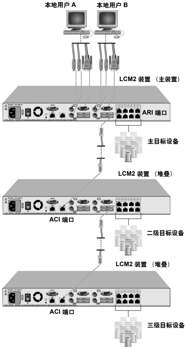
图 2.4：含堆叠装置的 LCM2 装置配置
