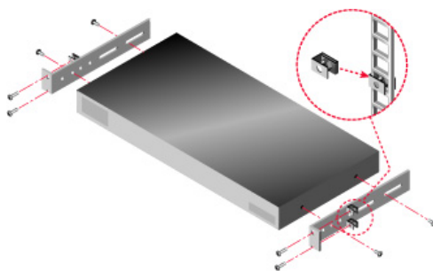
图 2.2：水平安装装置
