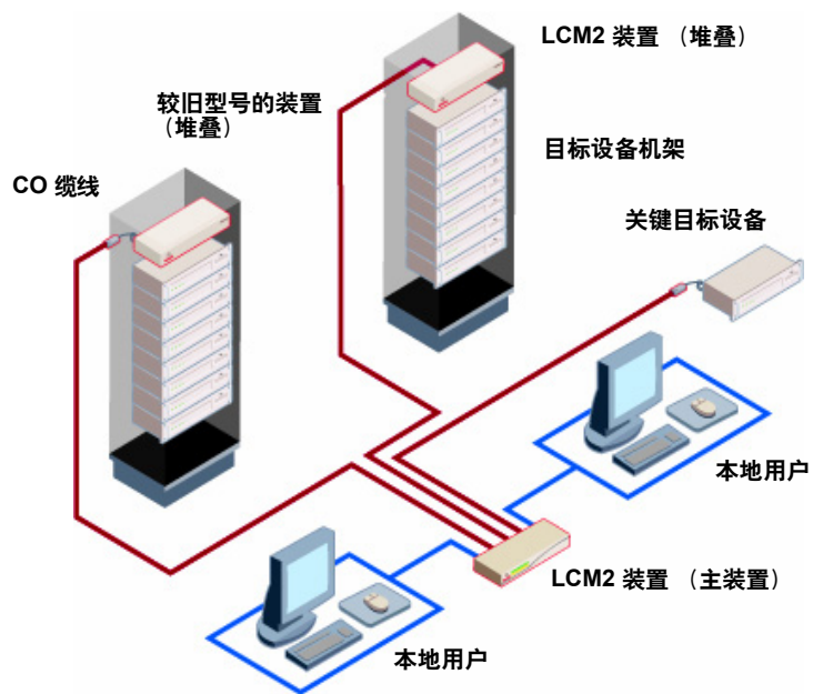
图 1.3: LCM2 装置配置示例
