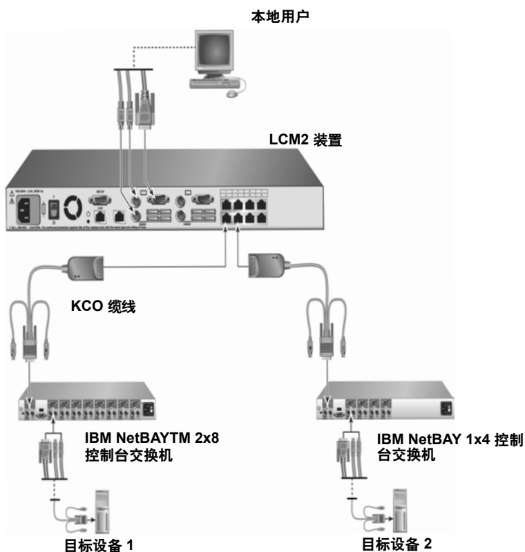
图 2.5：含有较早型号的装置的装置配置
