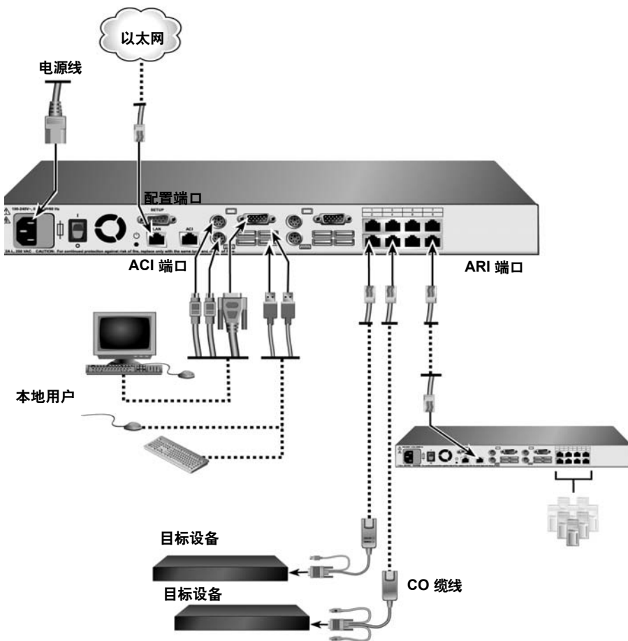
图 2.3: LCM2 装置基本配置
