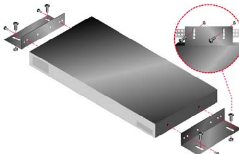
图 2.1：垂直安装装置
