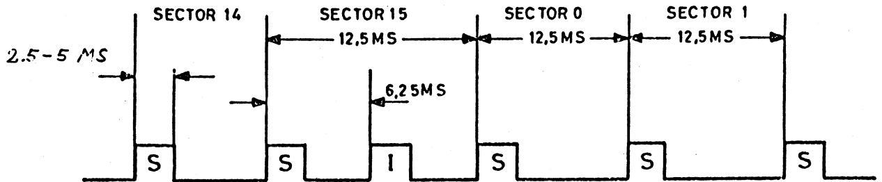
Abbildung 3.1.2.2 Index-Sektor-Impuls-Diagramm (hardsektorierte FlexyDisk)
