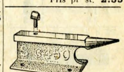
Instrumentmakarstöd № K 569. av stål, med avskrot. Storl. 26×8×8,5 cm. Vikt c:a 3 kg. Ett extra prima stöd av svenskt fabrikat. Pris pr st. 7:85
