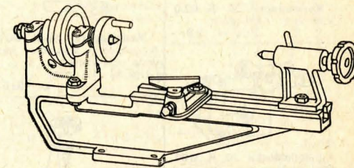
Svarv № K 590, med försättare № K 606 för handstål samt motdocka med cylindrisk, förskjutbar enkel dubb. Vikt c:a 2,2 kg. Pris kr. 36:65
