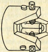
Chuck № K 600. med 3 st. var för sig ställbara härdade stålbackar. Gripes upp till 16 mm. Vikt c:a 200 gram. Pris kr. 12:50
