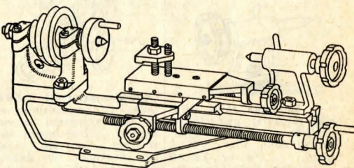
Svarv № K 592, lika svarv № K 591, men dessutom försedd med ledareskriv № K 611. Vikt c:a 3,2 kg. Pris kr. 63:75
