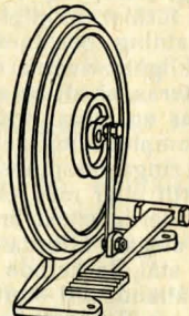
Fotdrift № K 613. med 3 st. hastigheter och en liten extra remskiva för låga varvtal och stor dragkraft. Diam. 300 mm. Vikt c:a 11 kg. Pris kr. 39:50 Svänghjul № K 614 m. extra prima kvalitet, graderad skiva för inställning, vevstake och pedal. Likaså förbättrad konstruktion. № K 613, men för montage i bänk. Utan ställning. Vikt c:a 8 kg. Pris kr. 33:75
