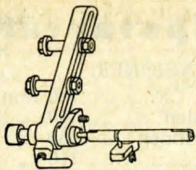
Hjulhållare № K 596. med hjultapp, koppling och kopplingsarm. Utan kugghjul. Vikt c:a 200 gr. Pris kr. 17:-
