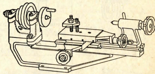
Svarv № K 591, lika svarv № K 590, men med korsupport № K 610 i stället för försättare. Vikt c:a 3 kg. Pris kr. 52:70
