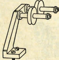
Remledarearm № K 595 med två brytullar. Att användas vid drift under bänk av svarv med automatisk matning, med eller utan oljetallrik. Vikt c:a 500 gram. Pris kr. 12:85
