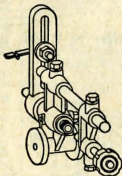
Delningsapparat № K 594. fästes på vertikalsliden eller på verktygsslid på vinkelhylla. Spindelnoson lika svarvens. Svarvens växel-hjul användas för delning. Kombinerad delning möjlig. Användes vid fräsning av kugghjul, gradering m. m. Utan kugghjul. Vikt c:a 800 gr. Pris kr. 39:50
