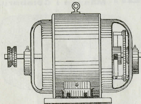
N:o 344. Motor för 220 volts växelström, att koppla direkt på ledningsnätet. Med ring- smörjningslager och ställbara borstar. Vikt c:a ett kilogram. Passande att draga mindre smärjelskivor m. m. Pris ..... 21.—
