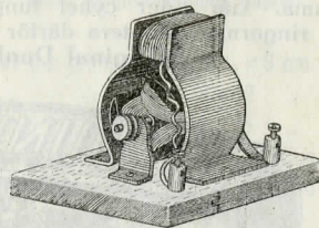
N:o 343. Motor för 2—4 volt, men kan den även kopplas till en vanlig belysningsledning om man kopplar den i serie med en glödlampa. Den trevligaste och nyttigaste leksak för pojkar. Pris ..... 5.75
